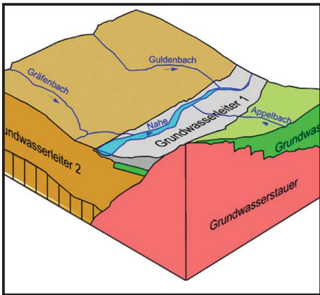
Erfassung hydrogeologischer Grundlagen Hydrologische Systemdarstellung
